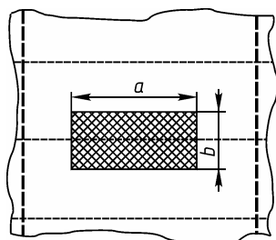
Рис.15.1.8-2. Площадка нагружения для ребра жесткости
