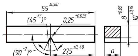
Рис. П10.2.8-2. Образец с V-образным надрезом для испытаний на работу удара КИ. a = (10 \pm 0,10) мм, a = (7,5 \pm 0,10) мм или a = (5 \pm 0,06) мм
